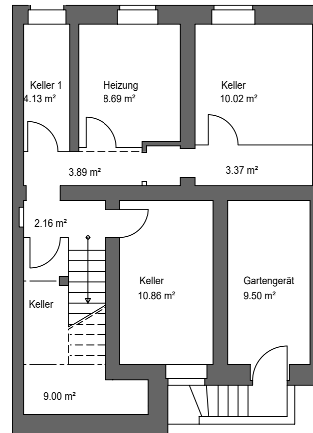
KELLERGESCHOSS
