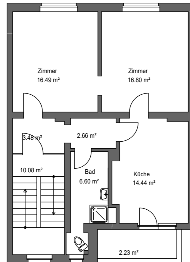
1. OBERGESCHOSS
