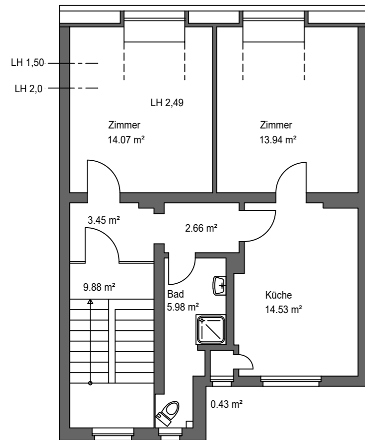
DACHGESCHOSS
